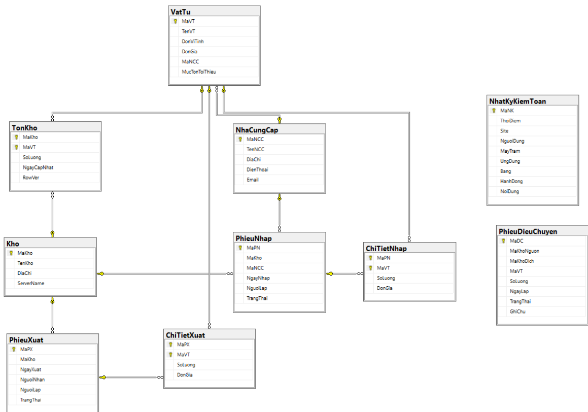
Hình II.1: Sơ đồ quan hệ do SSMS sinh tại site KHO_A — chín bảng nghiệp vụ và bảng nhật ký kiểm toán
